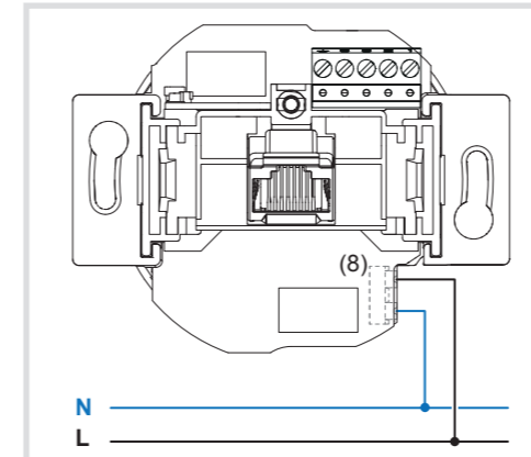
Bild 3: Anschluss Versorgungsspannung
